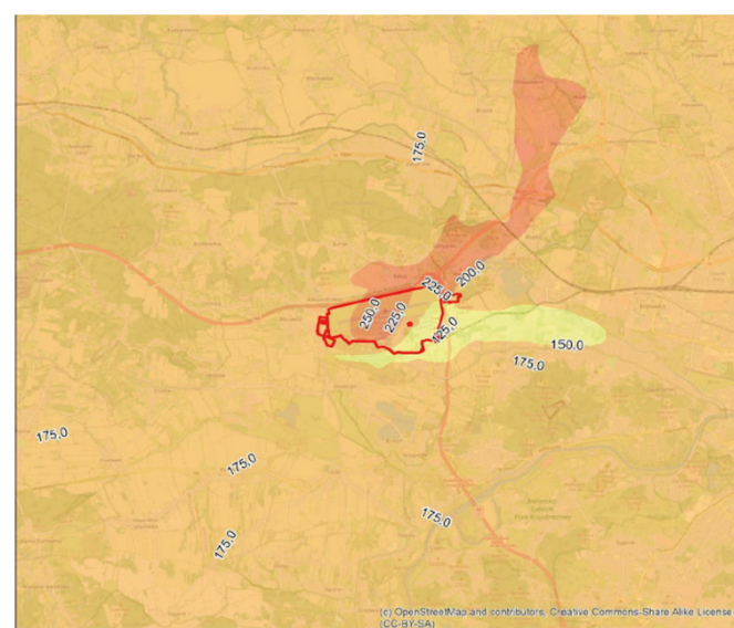
Rysunek VI. 67 Zmiana stężeń dwutlenku węgla dla horyzontu 2045 – Wariant Północny
