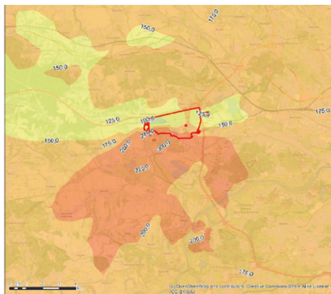
Rysunek VI. 68 Zmiana stężeń dwutlenku węgla dla horyzontu 2045 – Wariant Centralny
